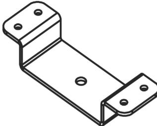
Herraje soporte ducto - Negro GAR840160PL00
