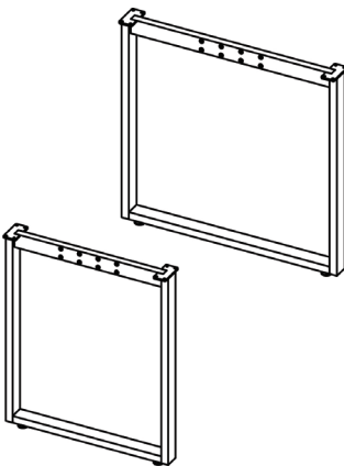
Pata lateral 60x9x72 cm - Aluminio texturizado GAR826060PT01
