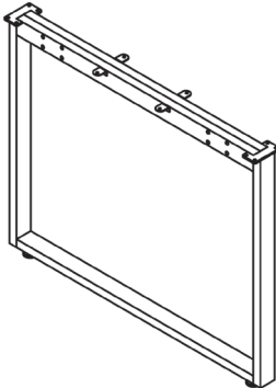
Pata central double run 90 x 9 x 72 cm - Aluminio texturizado GAR827090PT01
